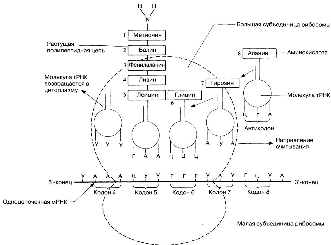
Рис. 23.30. Схематическое изображение процесса трансляции. Антикodon каждой отдельной молекулы аминокислот-тРНК спаривается с комплементарным ему кодоном мРНК на рибосоме. В изображенном здесь случае за этим последует образование пептидной связи между лейцином и глицином и таким образом к растущей полипептидной цепи добавится еще одна аминокислота.
