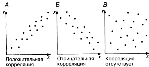
Рис. П.2.13. Типы корреляции; А — положительная корреляция; Б — отрицательная корреляция; В — корреляция отсутствует.
