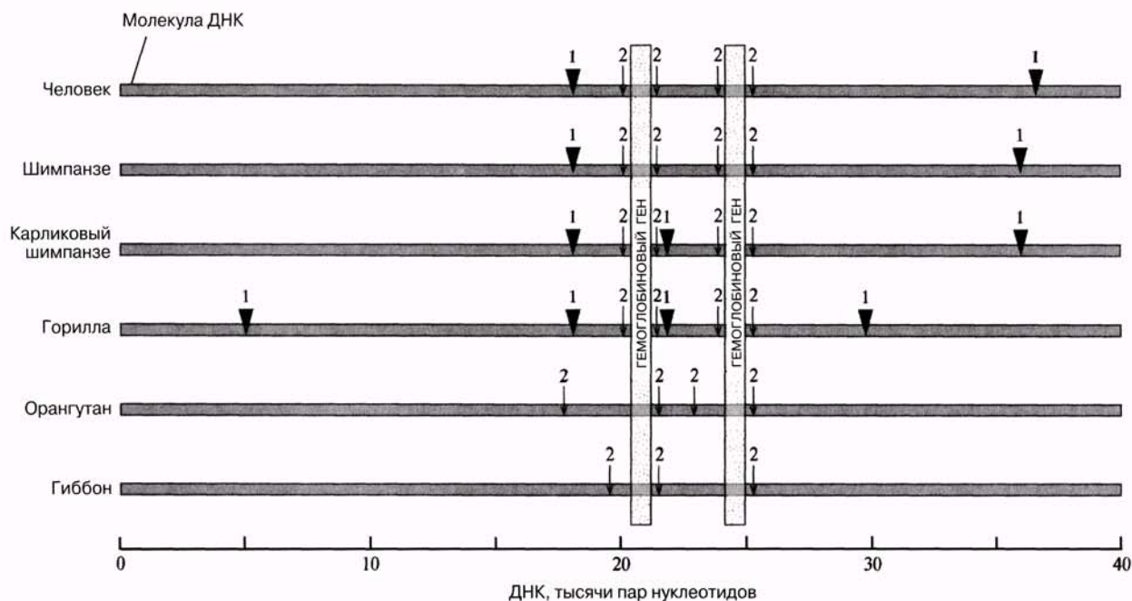
Рис. 25.3. Использование рестриктаз для разрезания ДНК и получения рестрикционных фрагментов разной длины. На этом рисунке участок ДНК, который содержит два гемоглобиновых гена разных приматов, обрабатывали двумя рестриктазами. Фермент 1 обозначен знаком ▼, фермент 2 — знаком ↓. Фермент 1 разрезает ДНК человека на два фрагмента, а фермент 2 — на пять фрагментов. Длины этих фрагментов, а также фрагментов, полученных при совместной обработке обоими ферментами, позволяют локализовать положение разрезов (сайтов рестрикции) относительно друг друга. На основе этих данных строят «рестрикционную карту», которая изображена на схеме. Чем больше рестриктаз используется для построения карты, тем более детальной она получается. Обратите внимание на то, что чем ближе родство между видами, тем более сходны их ДНК и расположение в них сайтов рестрикции. [Схема построена на основе рис. 7–4, с. 294, Molecular biology of the cell , 3rd ed., B. Alberts et al. (1994) Garland.]
