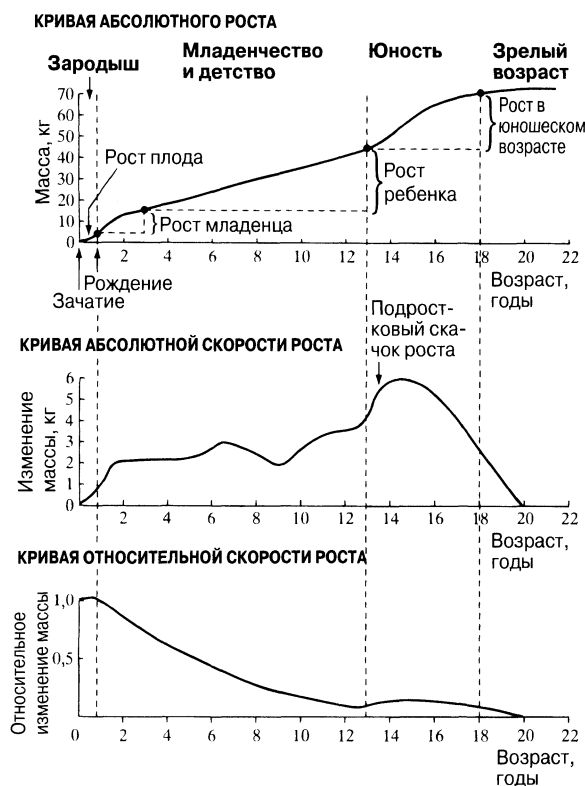
Рис. 22.6. Три типа кривых роста для человека.
