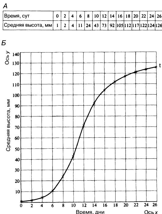
Рис. П.2.2. А. Два ряда данных: средняя высота проростков овса и продолжительность их роста. Б. График зависимости между средней высотой проростков овса и продолжительностью роста.
