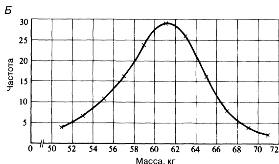
Рис. П.2.4. А. Представленная в виде таблицы численность 18-летних мужчин в каждом классе массы по 2 кг. Б. Графическое изображение данных из табл. А дает кривую нормального распределения.
