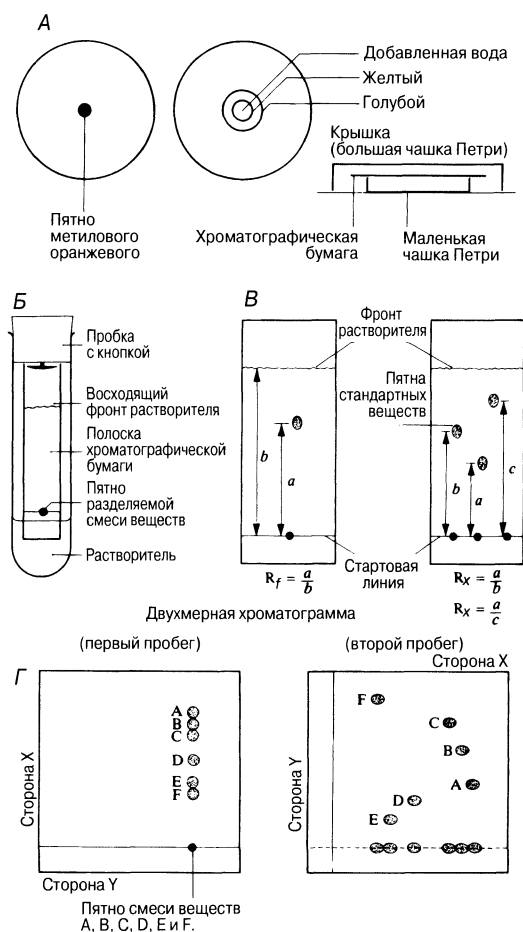
Рис. П.1.6. Методы хроматографии.
