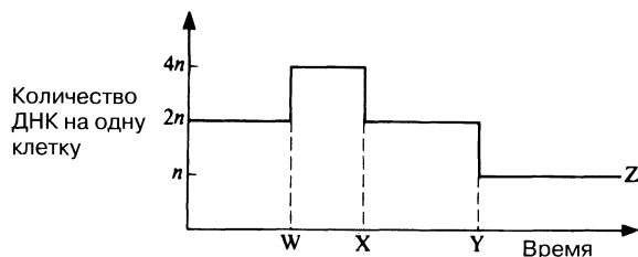
Рис. 23.15. График, который следует использовать при выполнении задания 23.1.
