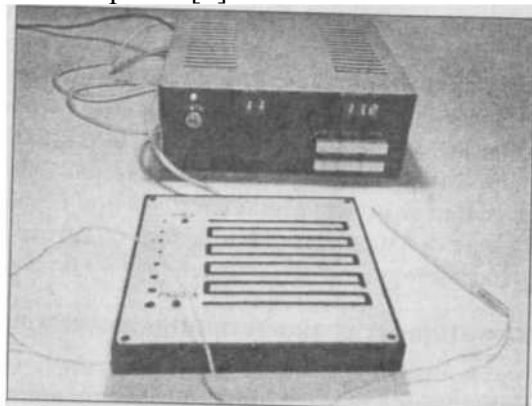
Рис. 13. Прибор для измерения состояния мышечной системы человека при стрессе (тремометр)
